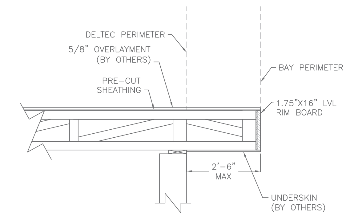
SECTION 6-A SCALE: 1/2"=1'-0"
